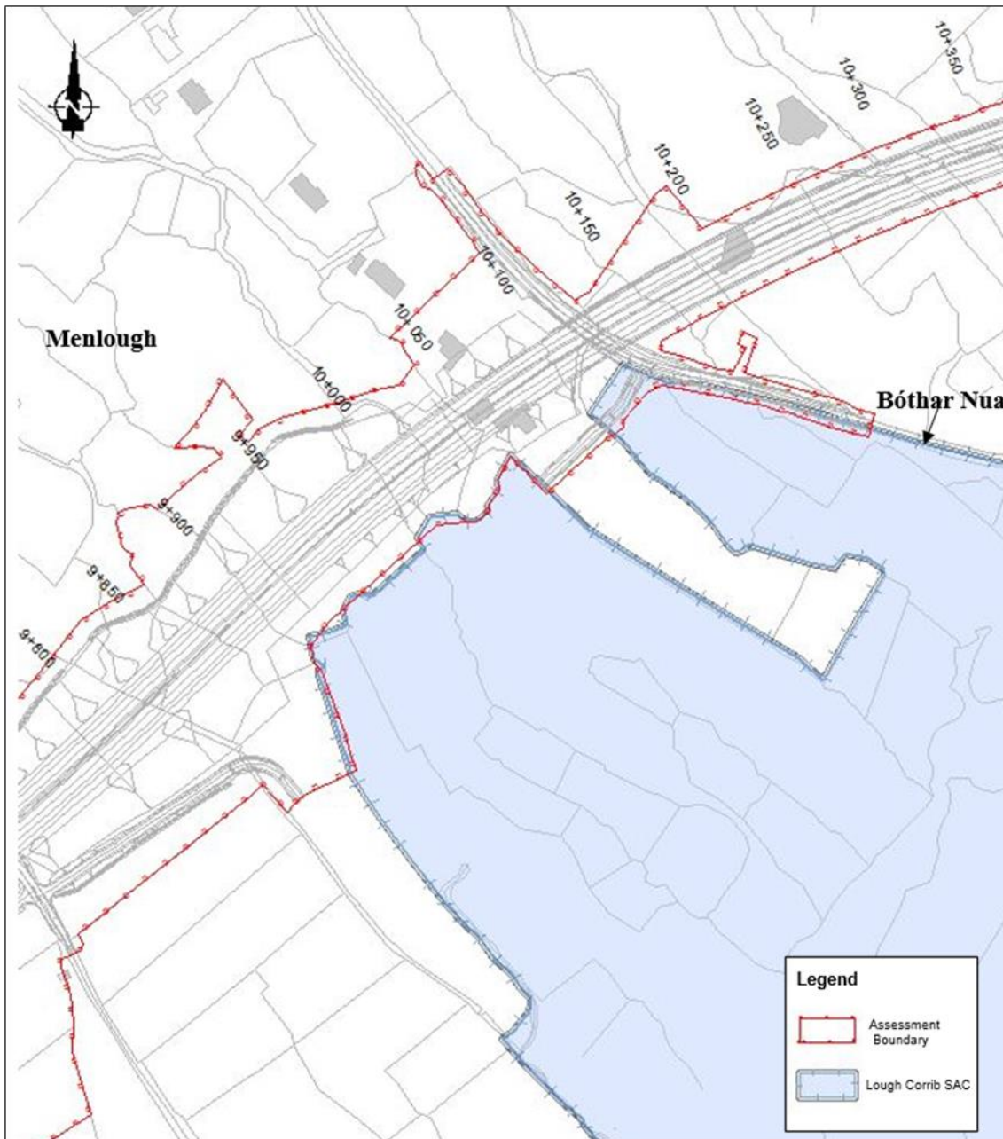
Pláta 2.5 Tionscadal Ch. 9+850 go dtí Ch. 10+150
