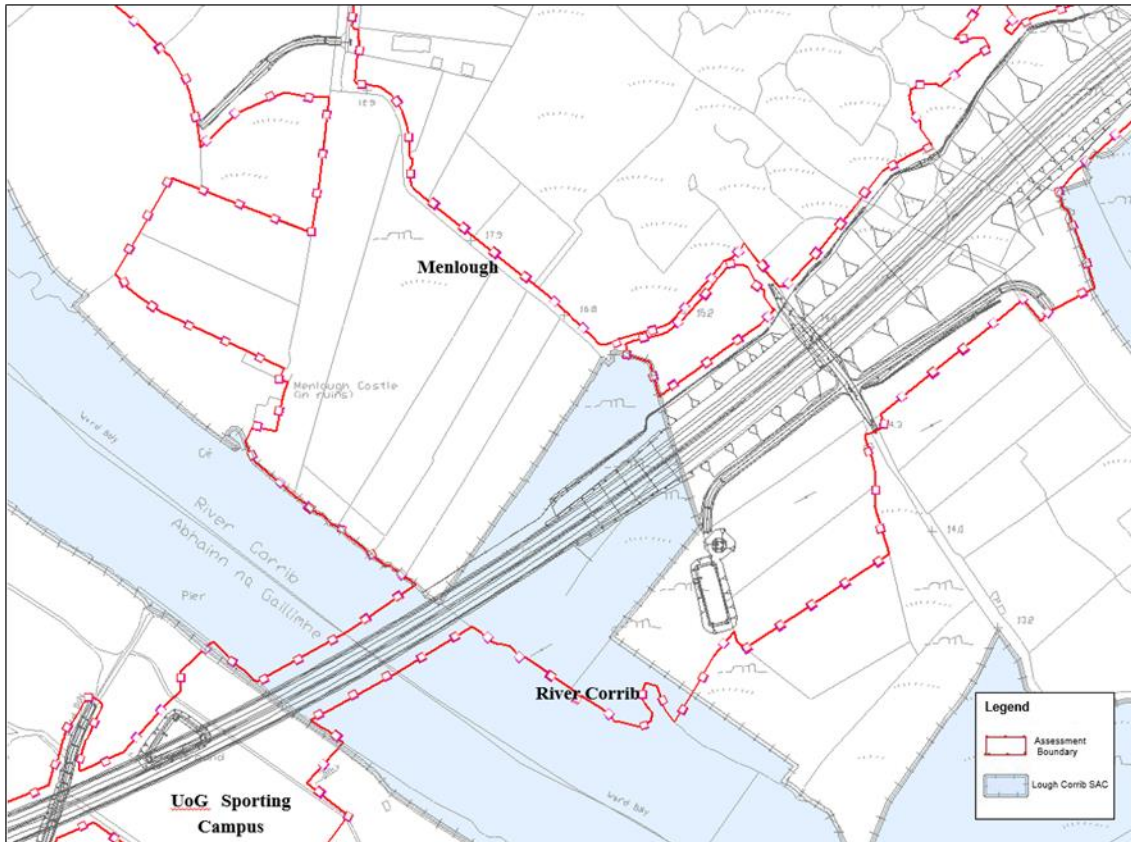
Pláta 2.4 Tionscadal Ch. 9+250 go dtí Ch. 9+550
